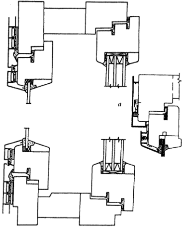
Рисунок 10 — Пример оконного блока раздельной конструкции (вертикальное сечение) с алюминиевыми облицовочными профилями
