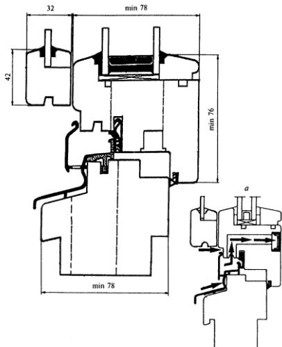
"Рисунок 1. Примеры конструктивных решений оконных блоков спаренной конструкции (основной и нижний притворы)"
