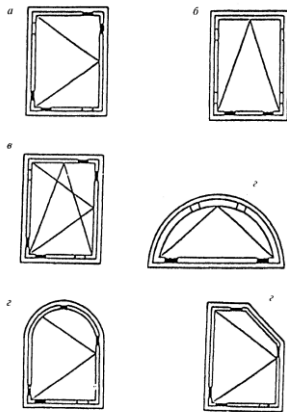
Виды открывания оконных блоков: а – поворотное (распашное); б – откидное; в – поворотно-откидное; г – установка подкладок в фигурных оконных блоках
