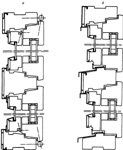
Рисунок 11 — Примеры горизонтального ( a ) и вертикального ( б ) сечений оконного блока спаренной конструкции с алюминиевыми облицовочными профилями
