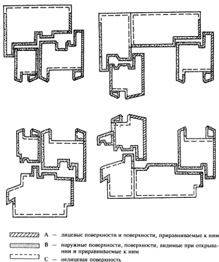
Рисунок 8 — Примеры определения видов поверхностей деталей
