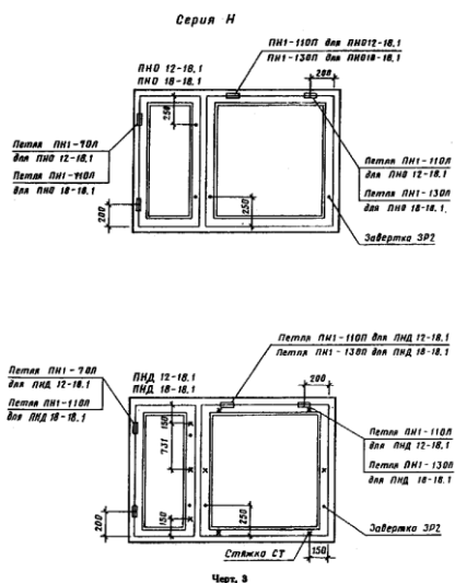
"Примеры расположения приборов в окнах. Серия Н. Чертеж 3. Приложение 4 (рекомендуемое)"
