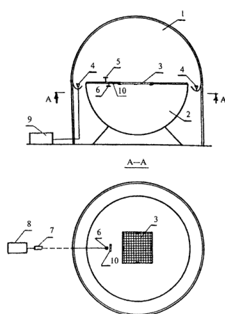
1 – источник диффузного света; 2 – светомерная камера; 3 – проем с опорной решеткой; 4 – осветительные приборы источника света; 5 – наружный фотозлемент; 6 – внутренний фотозлемент; 7 – переключатель фотозлементов; 8 – микроамперметр или гальванометр; 9 – регулятор напряжения осветительных приборов; 10 – экран фотозлемента от прямого света источника
