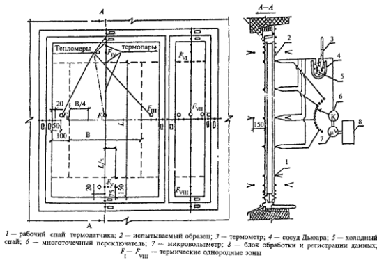
Рисунок 2 — Схема размещения термопар и тепломеров на образце оконного блока
