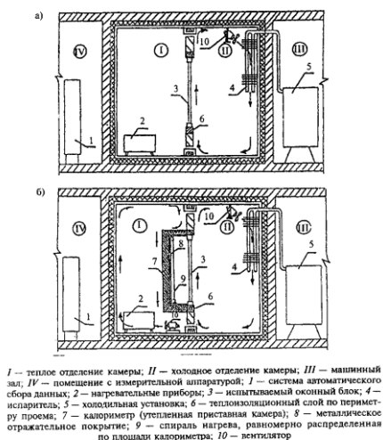
Рисунок 1 – Схемы климатической камеры для проведения испытаний: а) при измерении тепловых потоков при помощи термометров, б) с помощью приставной калориметрической камеры
